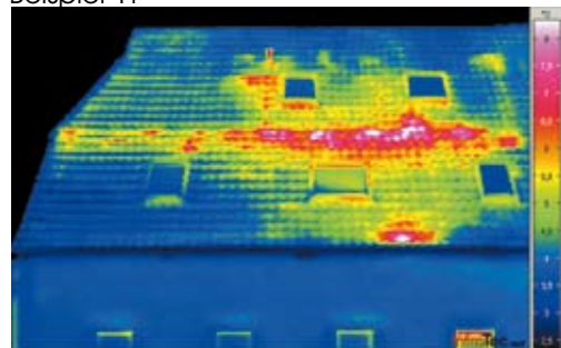
fehlerhafte Dachdämmung
